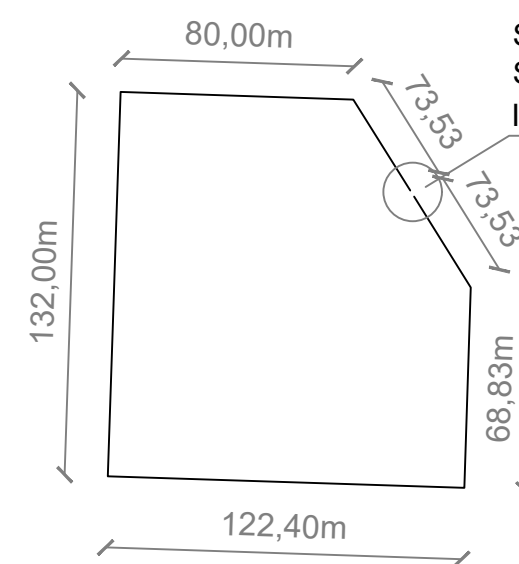
DETALLE 2 ESC 1:500
