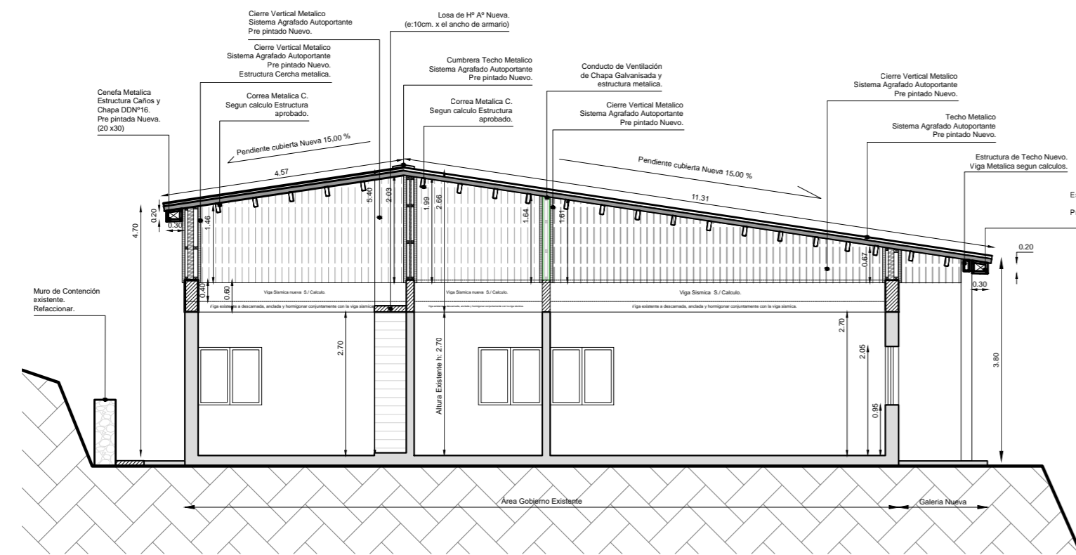
Corte 1 - 1
