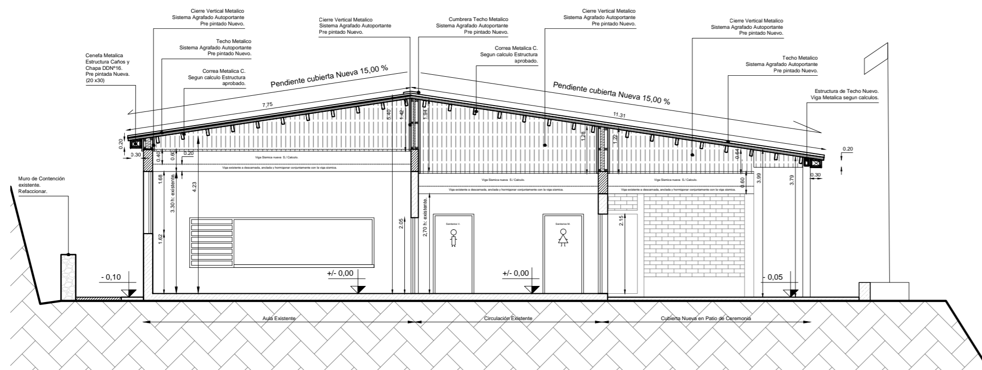
Corte 3 - 3
