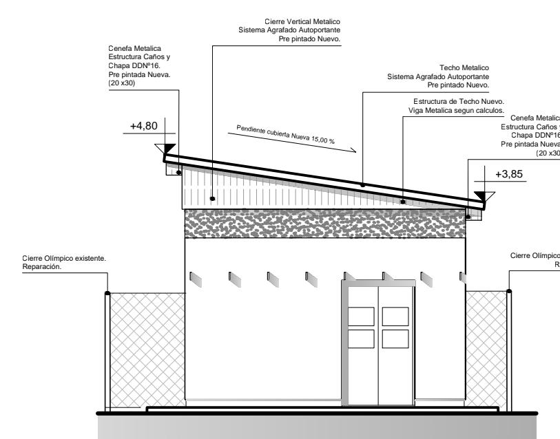
Fachada N. I. Sur-Oeste
