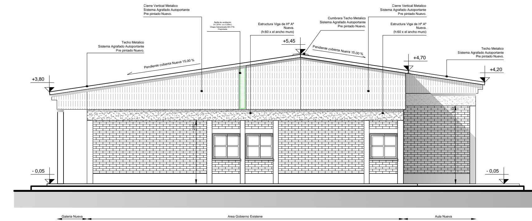
Fachada Nor-Oeste
