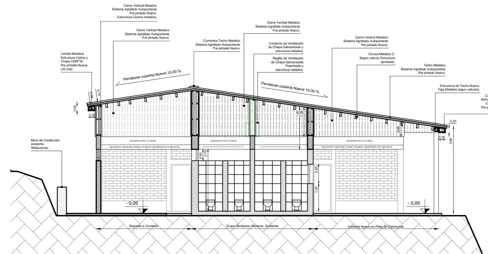
Corte 2 - 2
