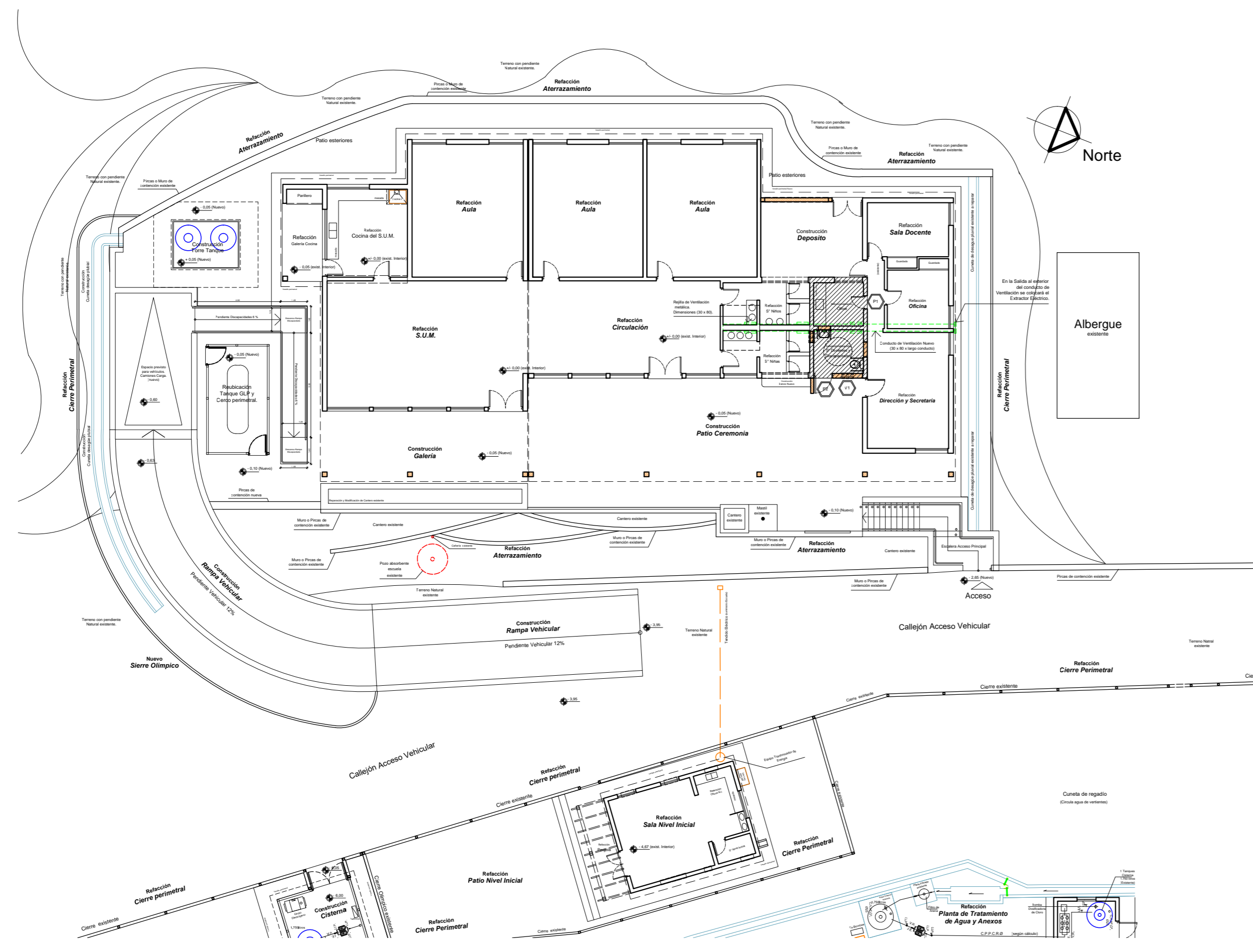
PLANTA - Esc. 1:200
