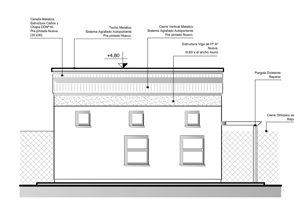
Fachada N. I. Nor-Este
