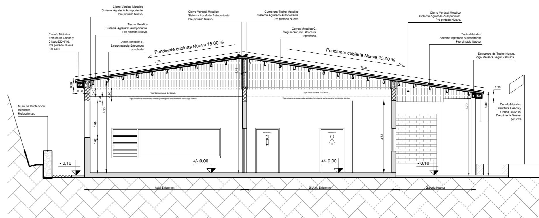
Corte 4 - 4
