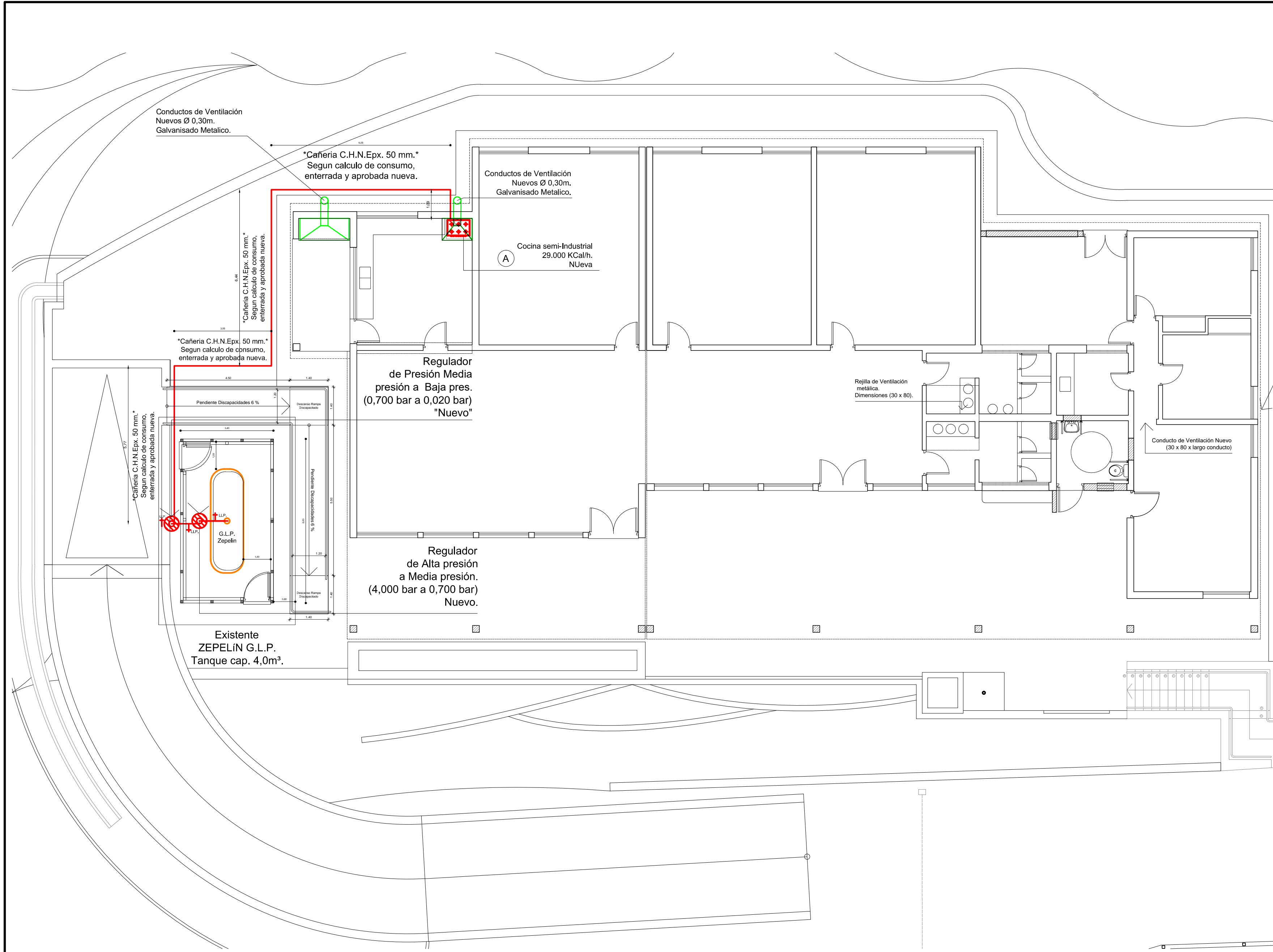
Plano Gas Nueva
