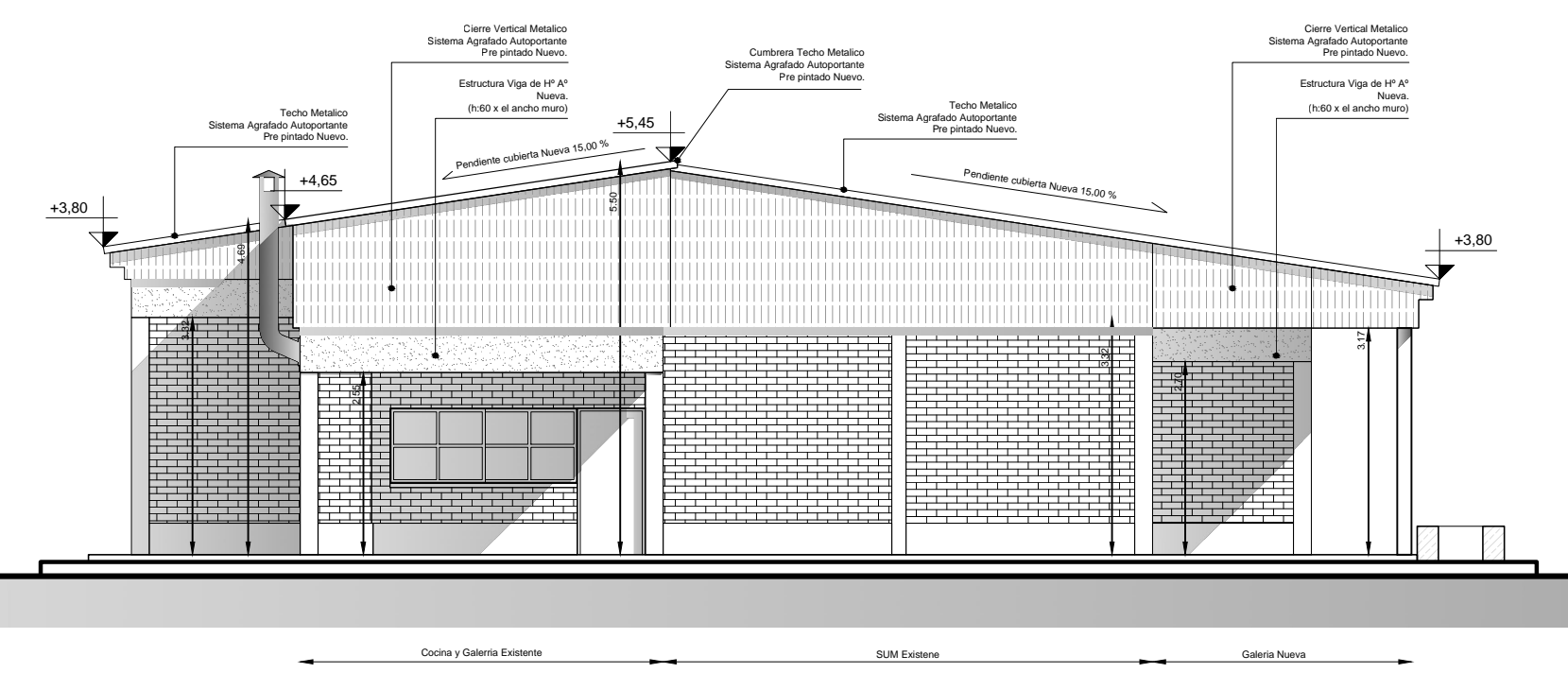
Fachada Sur-Este
