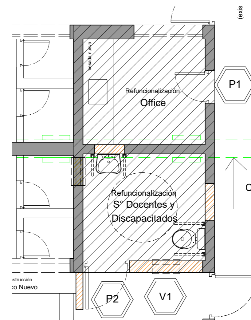
PLANTA - Sector a intervenir Esc. 1:50
